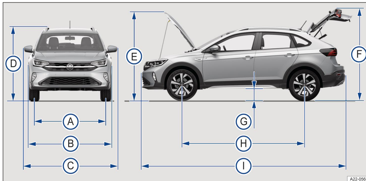
Фиг. 1 Размери на автомобила.
