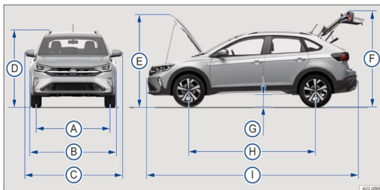
Фиг. 1 Размери на автомобила.
